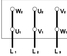
Şekil - 6: Δ Bağlantı
