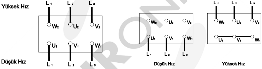
Şekil - 9: Çift Devirli Dahlender Sargılı Motor İçin Klemens Bağlantı Şeması
