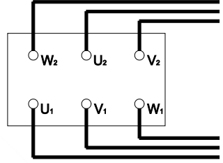
Şekil - 8: Y/Δ Bağlantı
