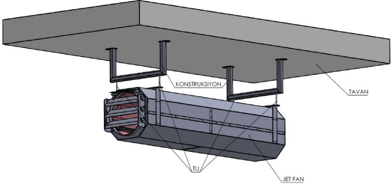
Şekil – 5: Aksiyal Tek Yönlü Jet Fan Bağlantı Şekli
