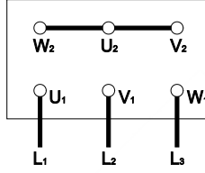
Şekil - 7: Y Bağlantısı
