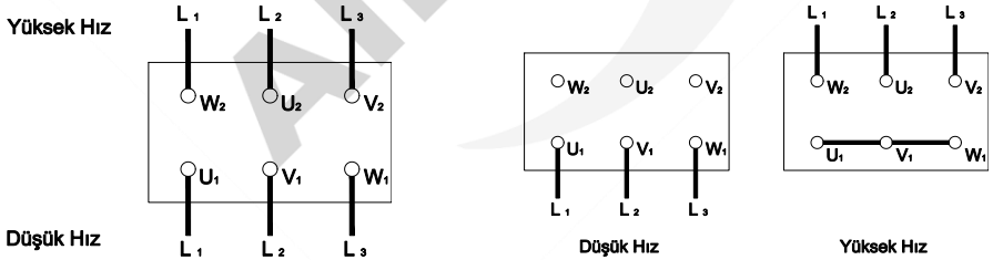
Şekil – 9: Çift Devirli Dahlender Sargılı Motor için Klemens Bağlantı Şeması
