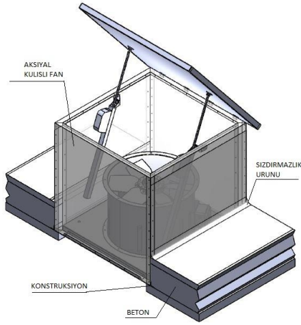
Şekil – 5: Aksiyal Kulisli Çatı Tipi Duman Egzoz Fan Bağlantı Şekli
